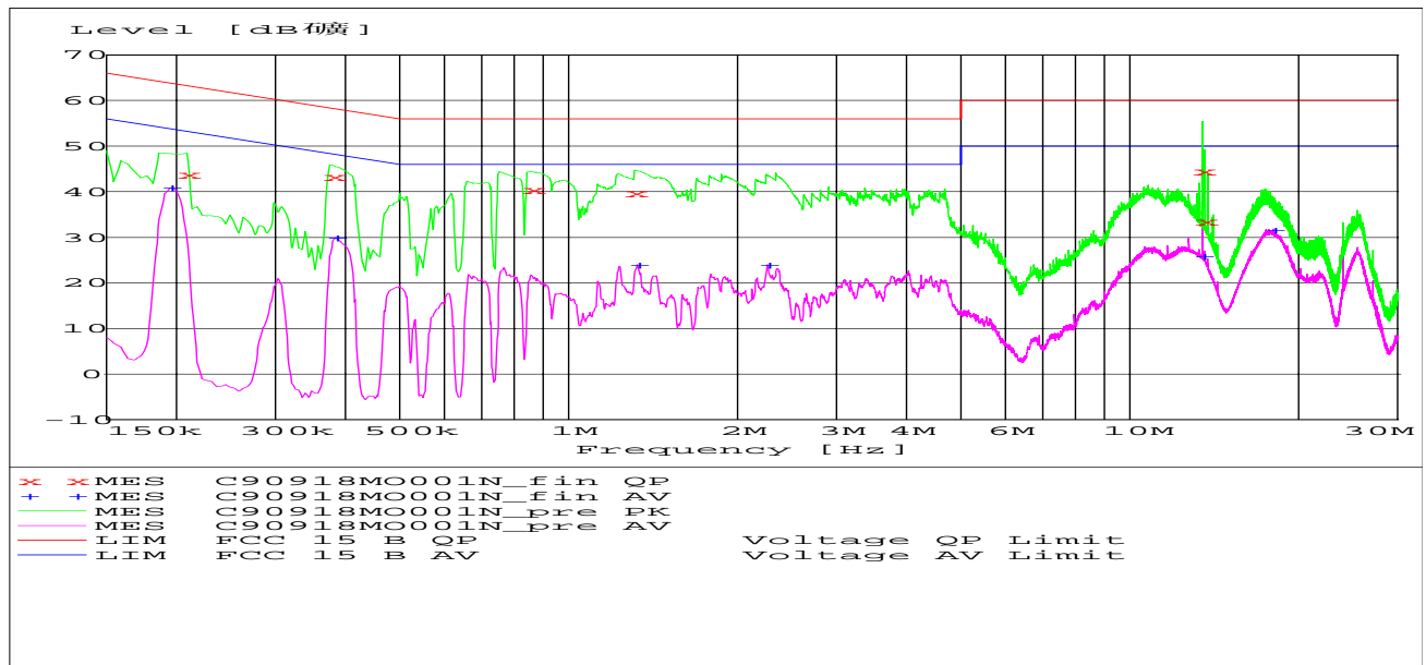
(Plot:N Phase)
