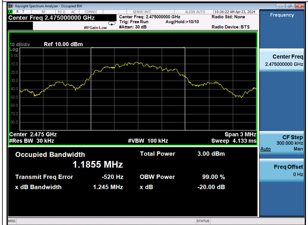
Test_Graph_GFSK_ANT1_2475_OBW
