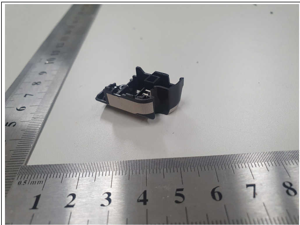
<LTE(MAIN) Antenna>
