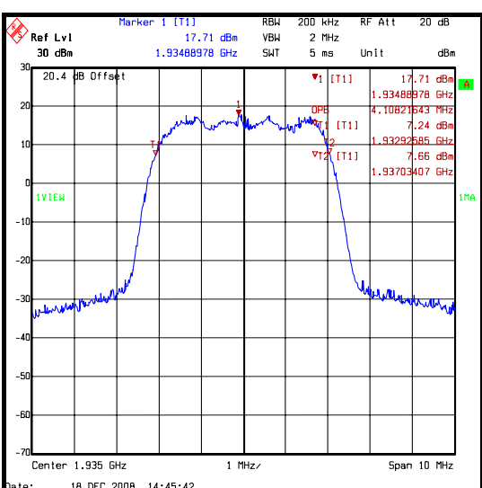
16-QAM (HSPA)
