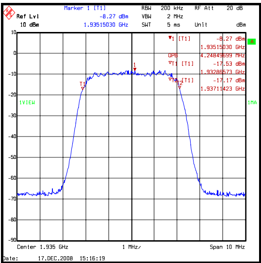
QPSK (UMTS)
