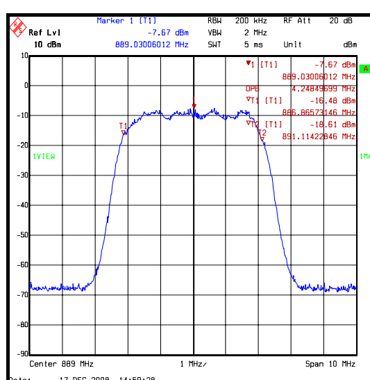
16-QAM (HSPA)
