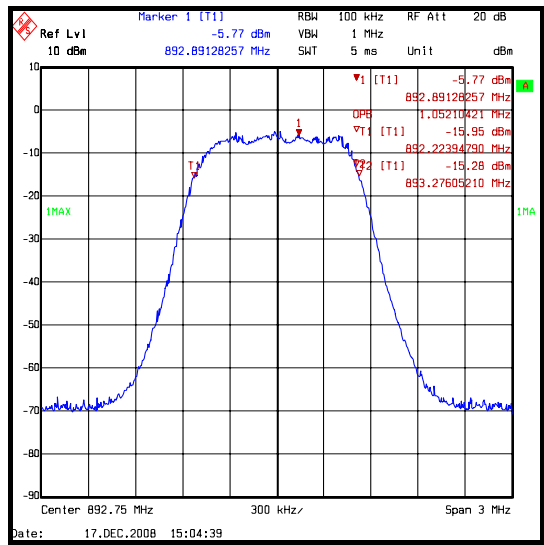
16-QAM (Ev-Do)
