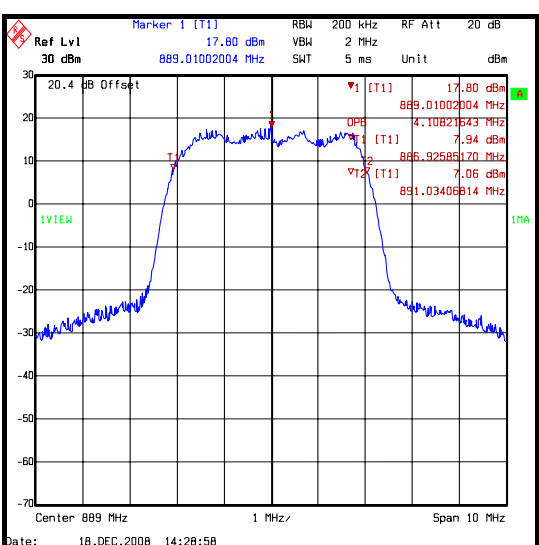
16-QAM (HSPA)
