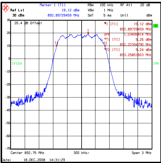
8PSK (Ev-Do)
