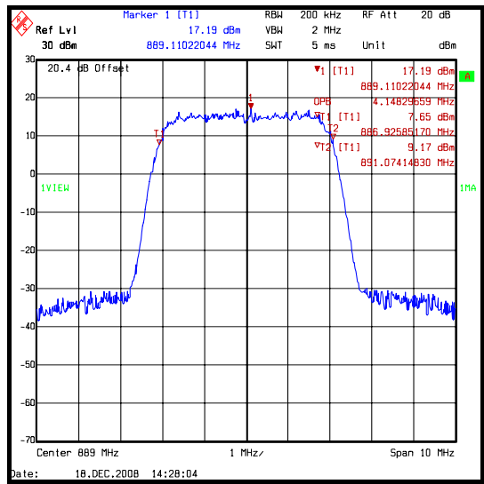
QPSK (UMTS)
