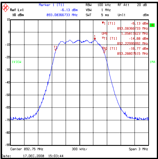
8PSK (Ev-Do)
