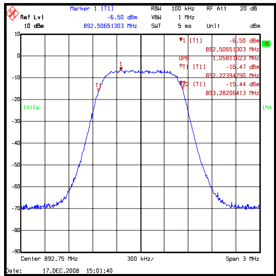
QPSK (CDMA)
