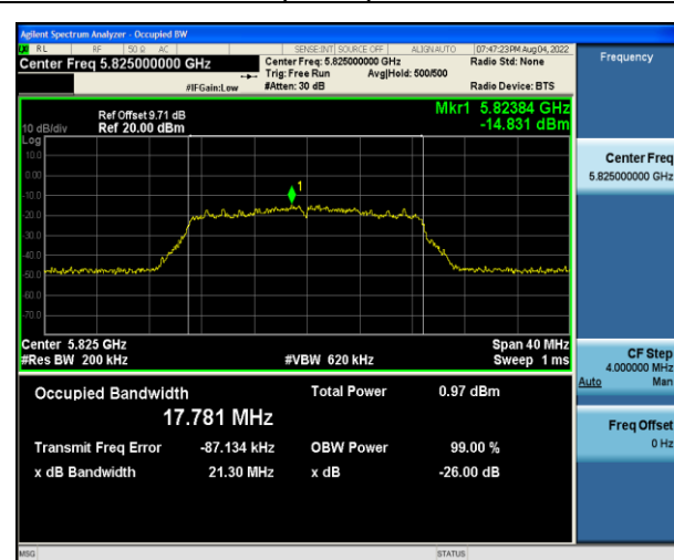
11ac(HT20) CH165
