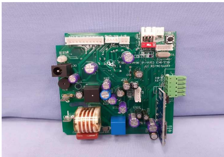
EUT Photo (16)
