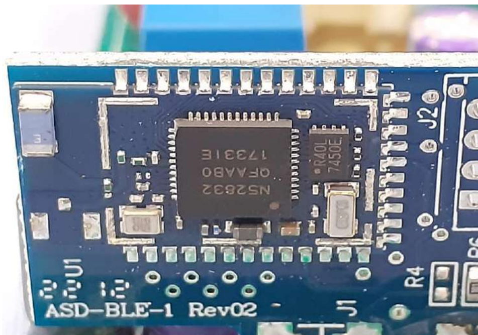
EUT Photo (12)
