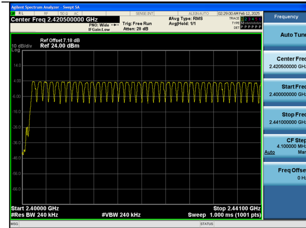
8DPSK (2.4 GHz - 2.441 GHz)
