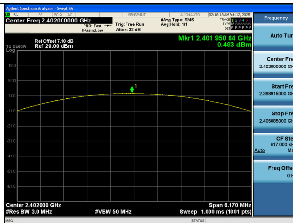
\pi/4 DQPSK : Peak Power (Ch. 0)
