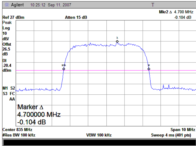
(Plot A: WCDMA 850MHz Channel = 4175)
