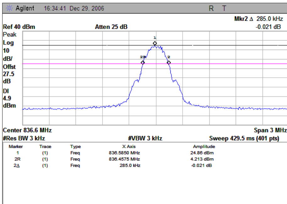
(Plot B: GSM 850MHz Channel = 190)
