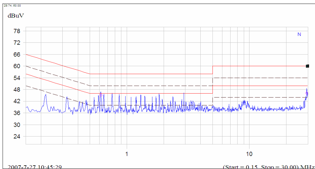
(Plot A: N Phase)
