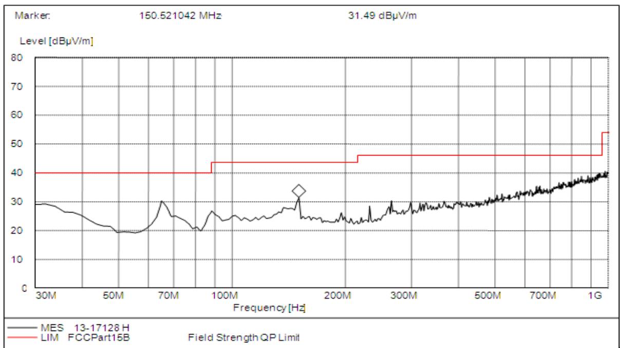
(Plot A: 30MHz to 1GHz, Antenna Horizontal)
