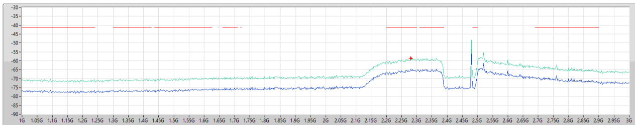
2.4-2.4835GHz_BT-LE(2Mbps)
