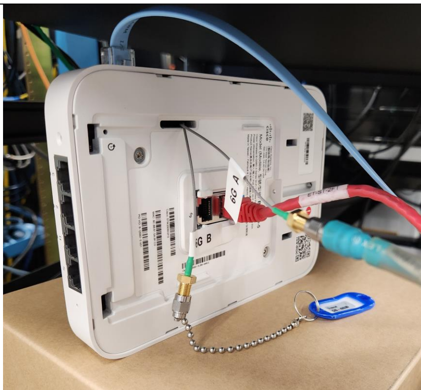
Title: AFC Setup - EUT
