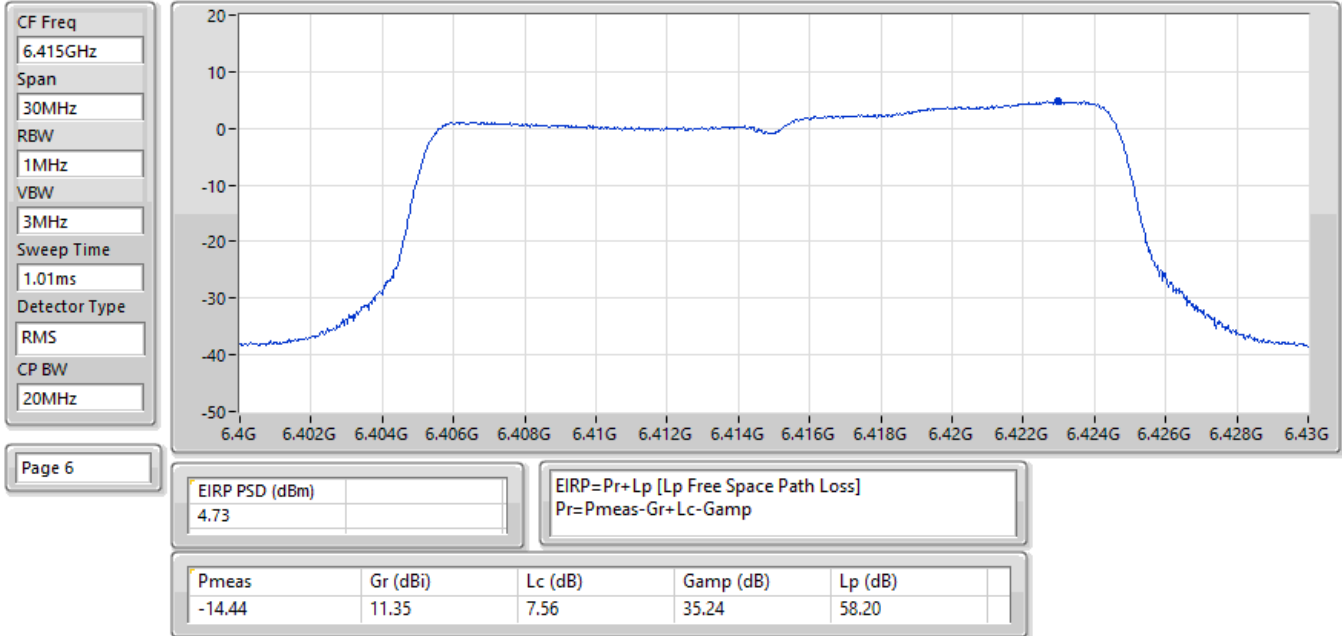
EIRP PSD;Band:6.2G;be20,BF;BWch:20MHz;Nss:1,(M0);Nant:2;Ch:6415MHz;TX
