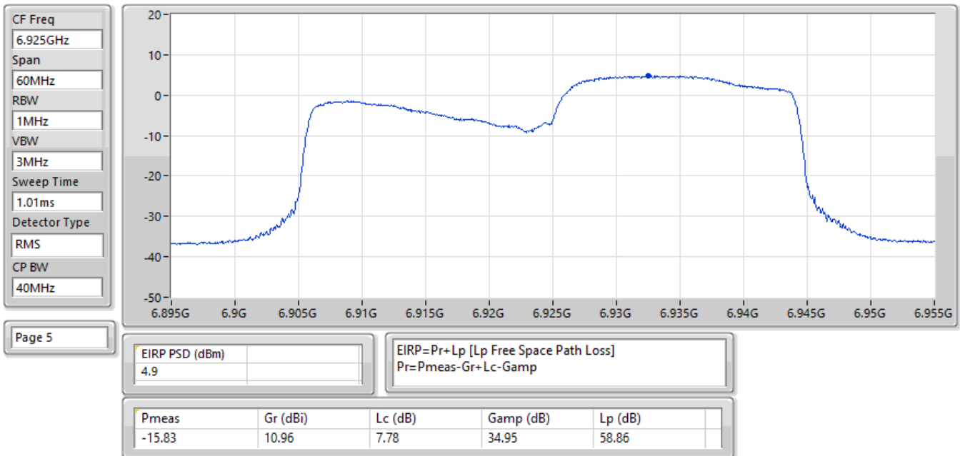
EIRP PSD;Band:7.0G;be40,BF;BWch:40MHz;Nss:1,(M0);Nant:2;Ch:6925MHz;TX
