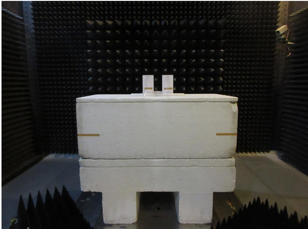
Radio1 Ant.27
