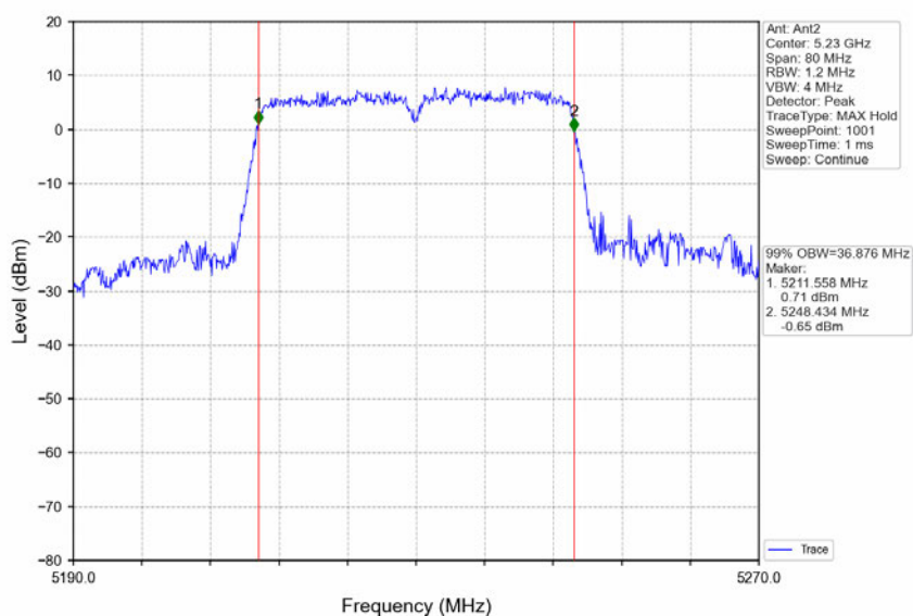
802.11n(HT40)_HCH_5230MHz_Ant2_NTNV
