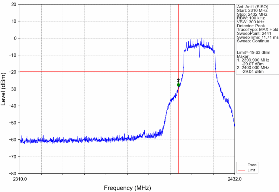
802.11n(HT20)_LCH_2412MHz_Ant1 (SISO)_NTNV
