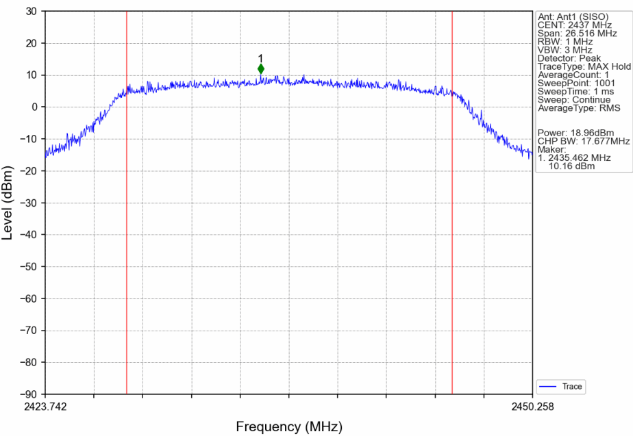
802.11ax(HEW20)_MCH_2437MHz_RU242_Left_Ant1 (SISO)_NTNV
