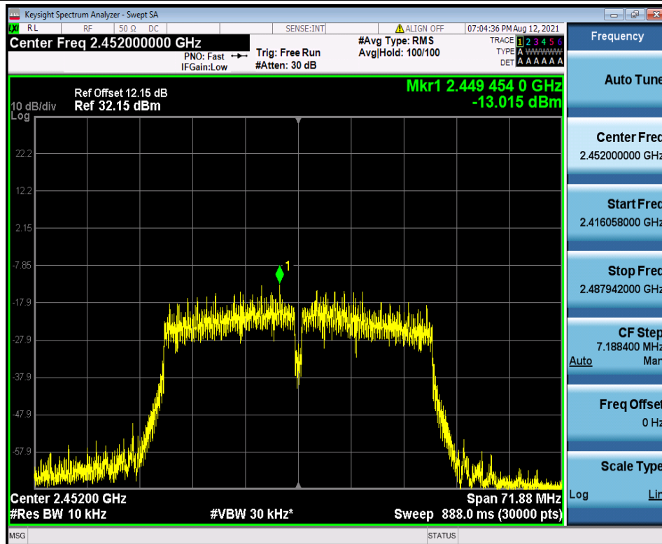
11N40SISO_Ant2_2452
