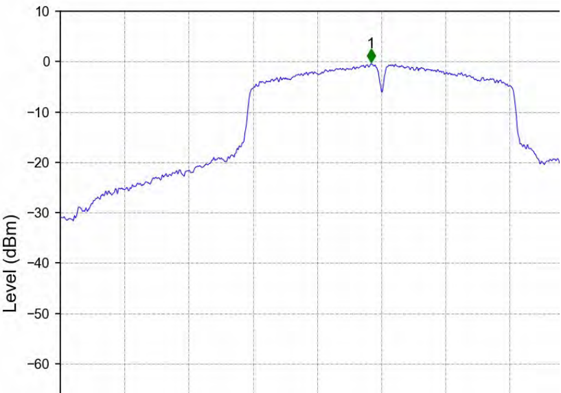
802.11a_HCH_5825MHz_Ant2_NTNV
