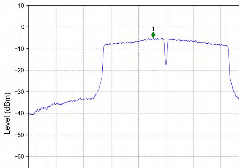
802.11ac(VHT40)_LCH_5755MHz_Ant2_NTNV
