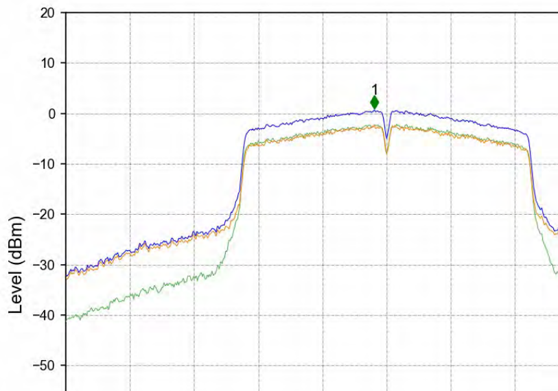
802.11n(HT20)_MCH_5785MHz_Ant1_NTNV
