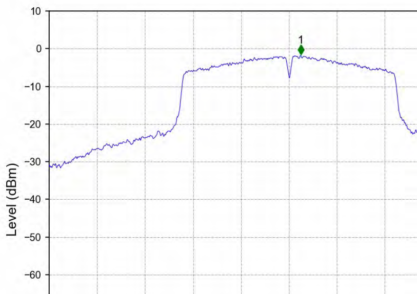
802.11n(HT20)_MCH_5785MHz_Ant1_NTNV
