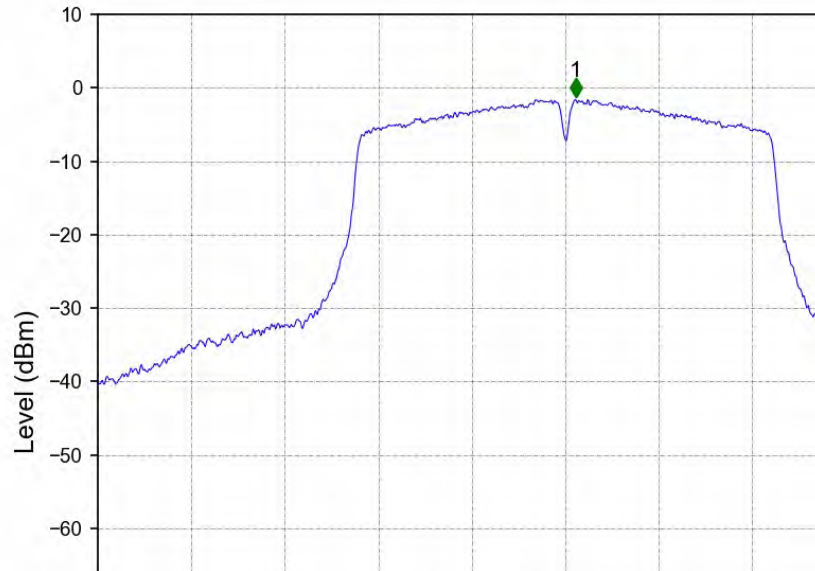
802.11n(HT20)_MCH_5785MHz_MIMO_NTNV
