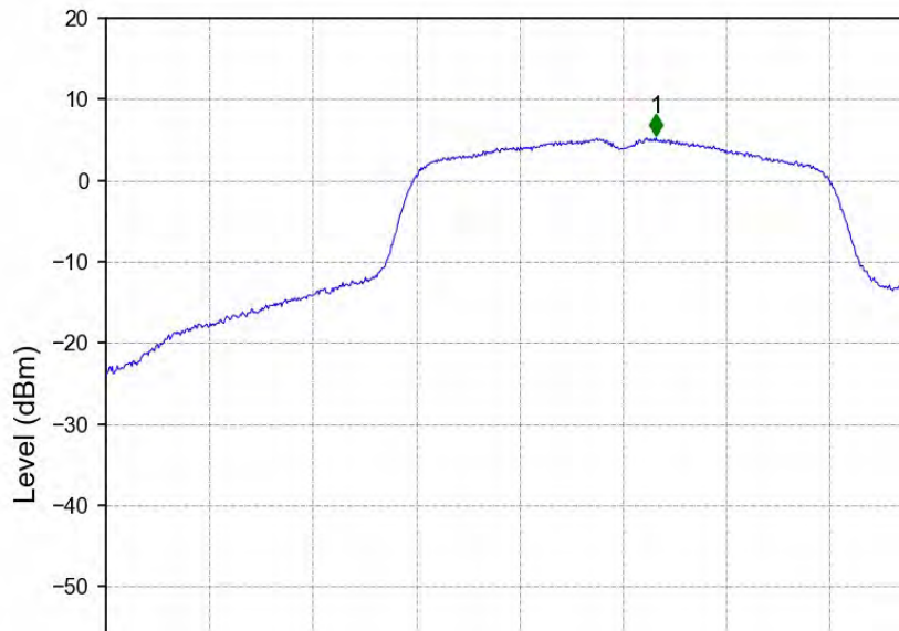
802.11a_MCH_5580MHz_Ant2_NTNV
