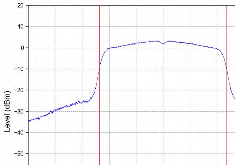
802.11n(HT20)_LCH_5260MHz_Ant2_NTNV
