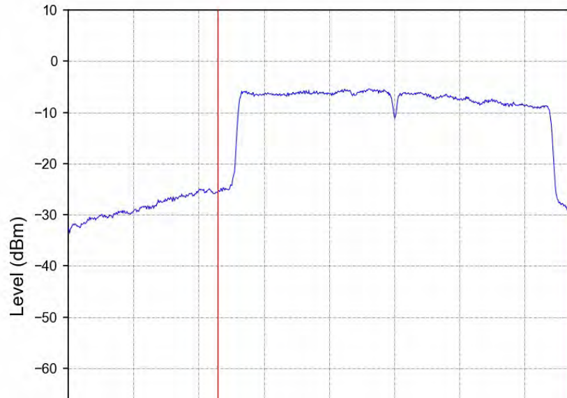
802.11ac(VHT80)_HCH_5610MHz_Ant2_NTNV
