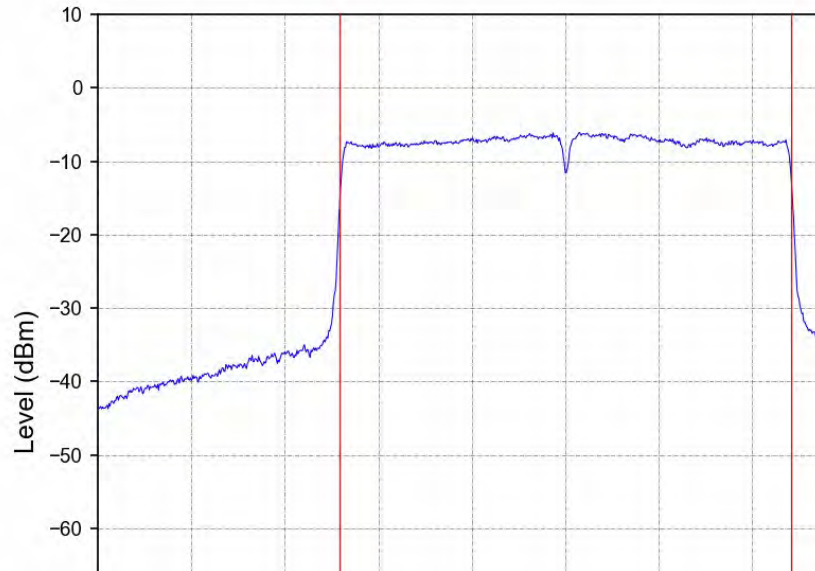
802.11ac(VHT80)_MCH_5210MHz_Ant2_NTNV
