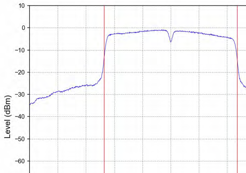
802.11n(HT40)_LCH_5510MHz_Ant2_NTNV
