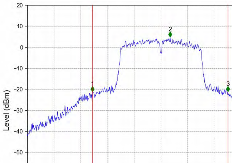
802.11ac(VHT40)_LCH_5270MHz_Ant2_NTNV
