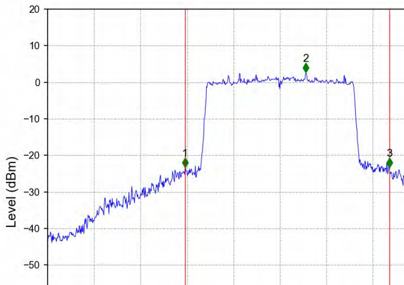
802.11ac(VHT80)_MCH_5210MHz_Ant2_NTNV
