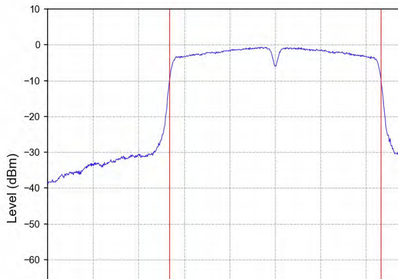
802.11n(HT40)_HCH_5795MHz_Ant2_NTNV
