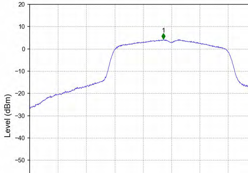
802.11a_LCH_5500MHz_Ant2_NTNV
