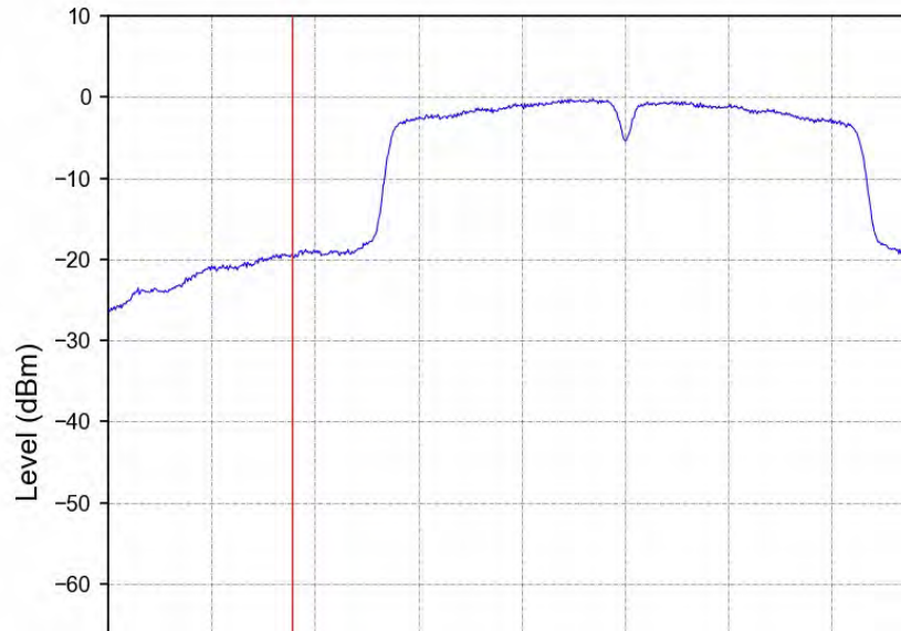
802.11n(HT40)_LCH_5755MHz_Ant2_NTNV
