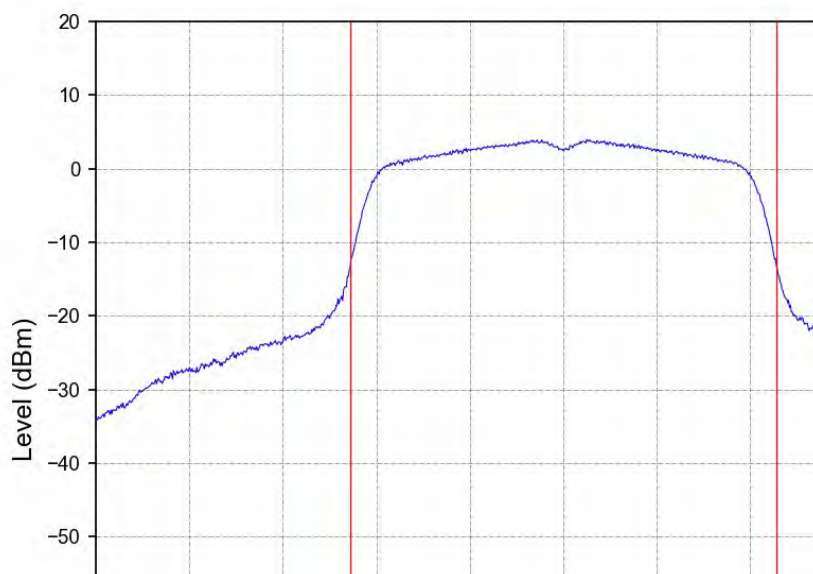
802.11a_MCH_5200MHz_Ant2_NTNV
