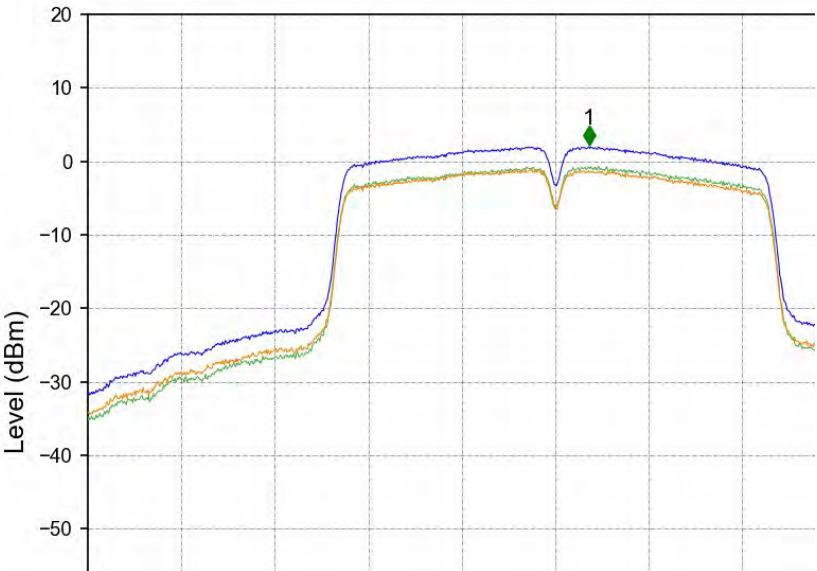
802.11n(HT40)_LCH_5510MHz_Ant1_NTNV
