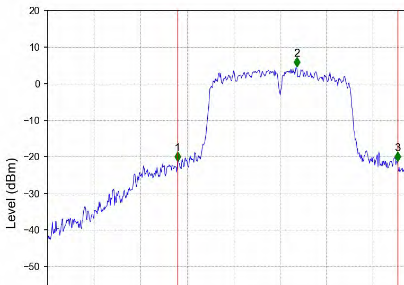
802.11ac(VHT40)_LCH_5270MHz_Ant2_NTNV
