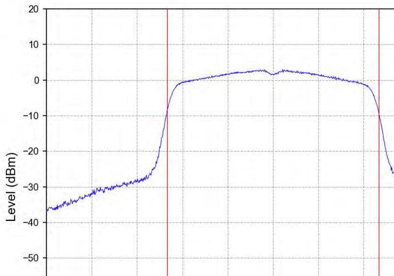
802.11n(HT20)_LCH_5180MHz_Ant2_NTNV
