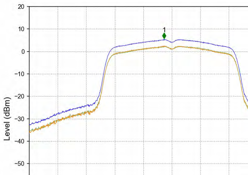
802.11n(HT20)_MCH_5200MHz_MIMO_NTNV
