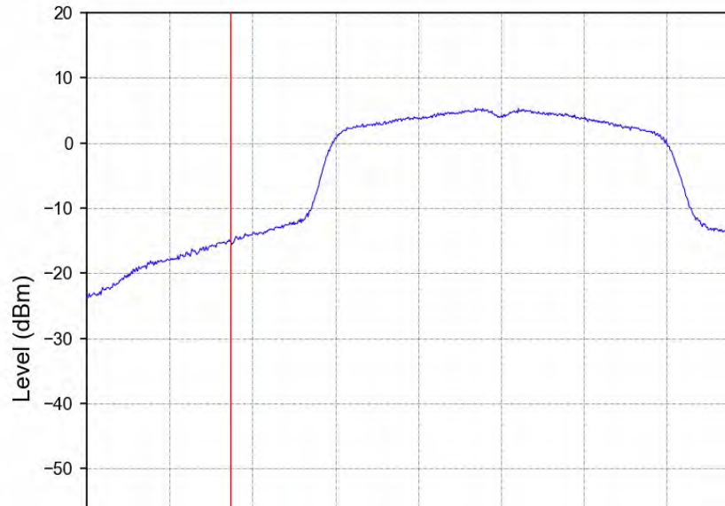
802.11a_MCH_5580MHz_Ant2_NTNV
