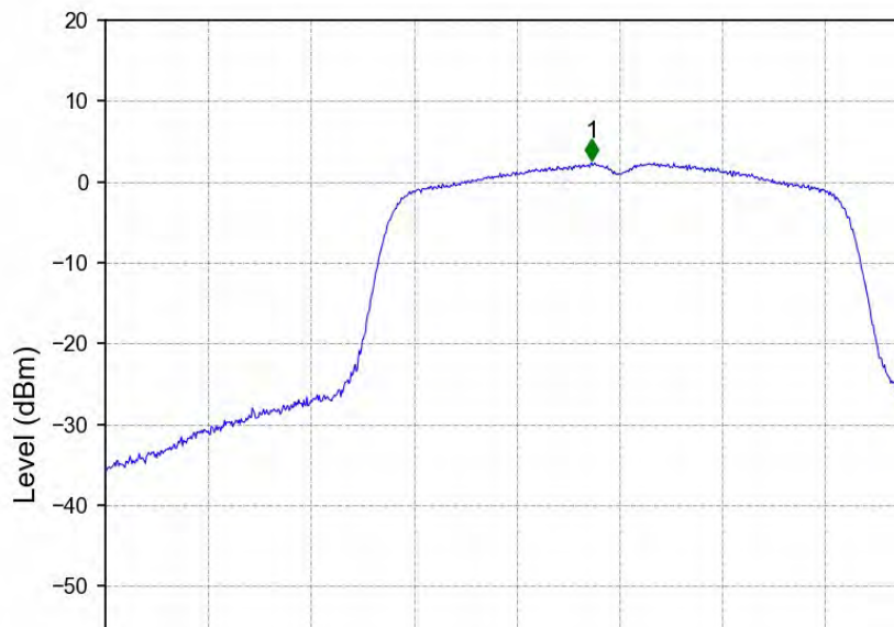
802.11n(HT20)_MCH_5200MHz_MIMO_NTNV
