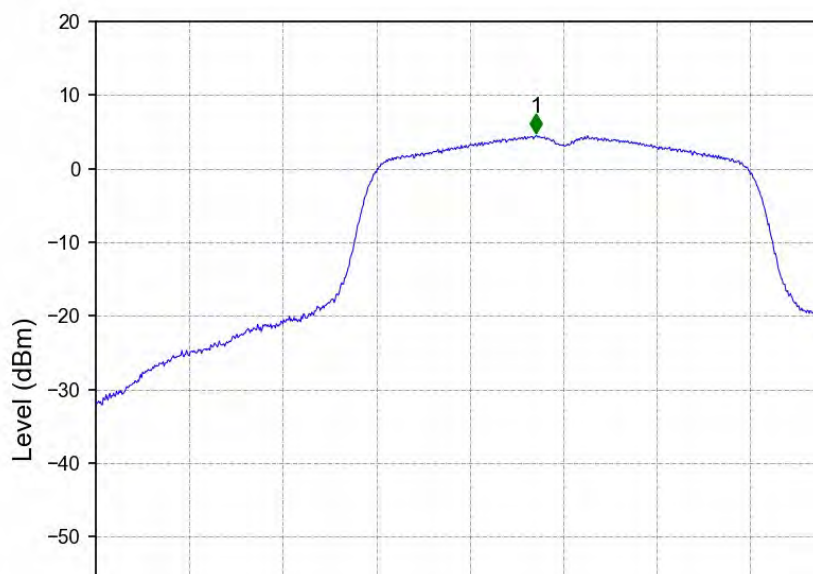
802.11a_MCH_5300MHz_Ant2_NTNV
