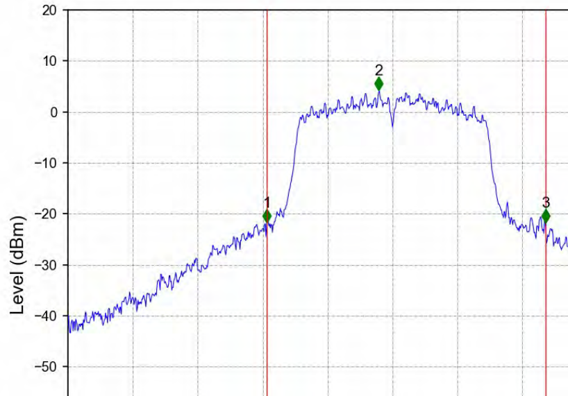
802.11n(HT20)_MCH_5200MHz_Ant2_NTNV
