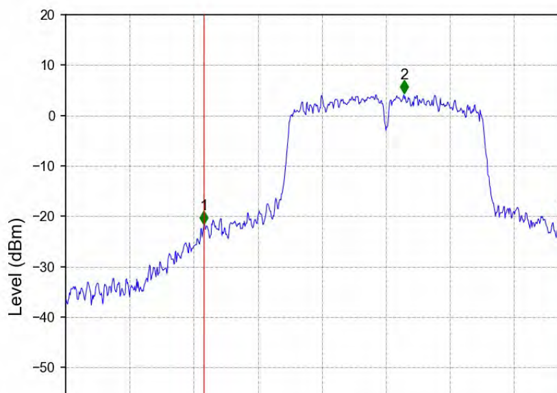
802.11n(HT40)_LCH_5270MHz_Ant2_NTNV
