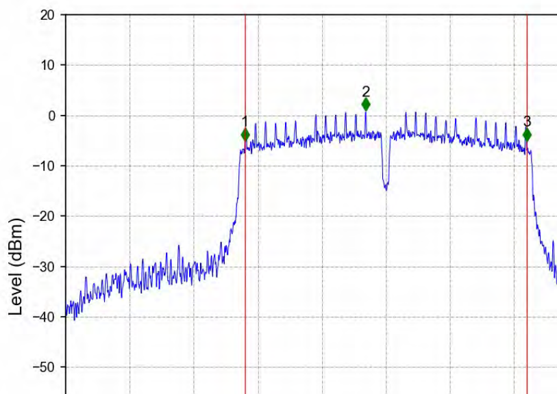
802.11n(HT40)_HCH_5795MHz_Ant2_NTNV
