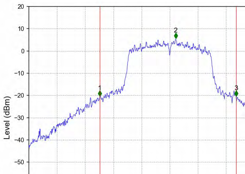
802.11n(HT20)_LCH_5500MHz_Ant2_NTNV
