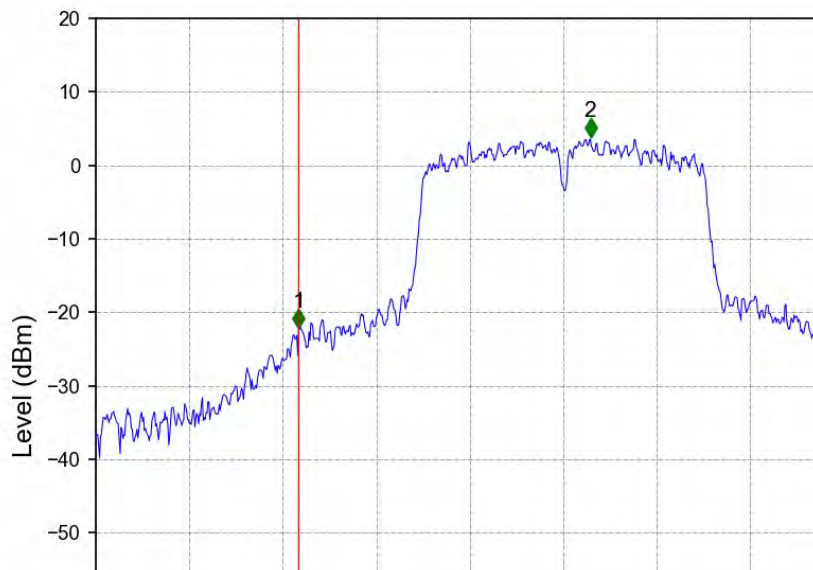
802.11n(HT40)_HCH_5230MHz_Ant2_NTNV
