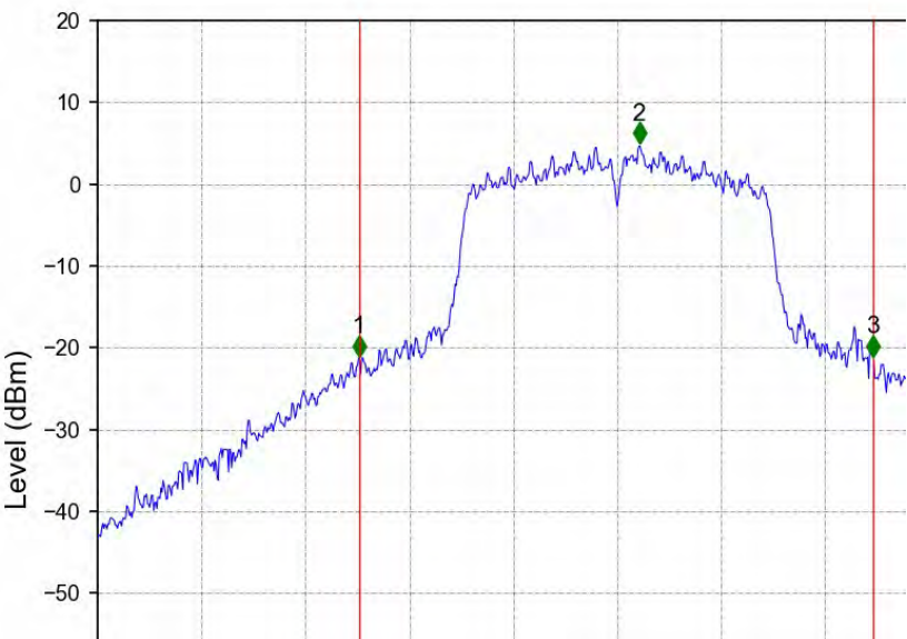
802.11n(HT20)_HCH_5320MHz_Ant2_NTNV
