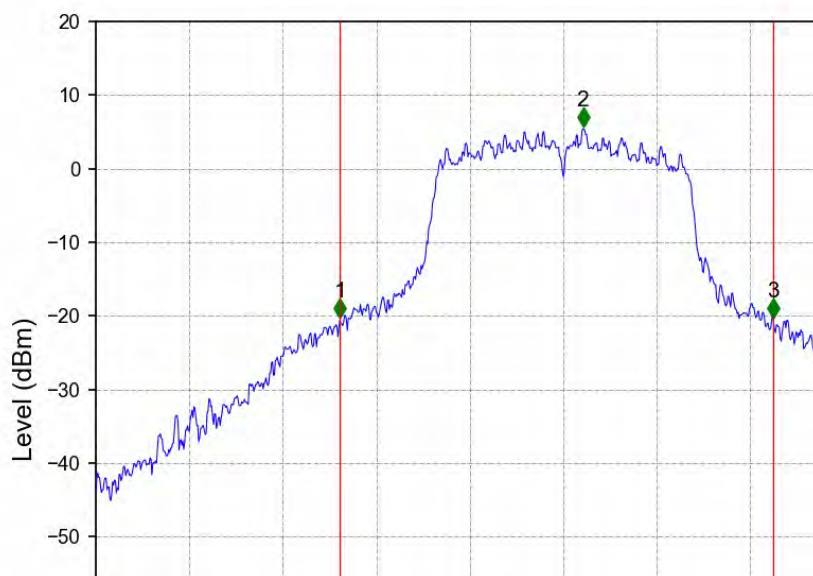
802.11a_LCH_5500MHz_Ant2_NTNV
