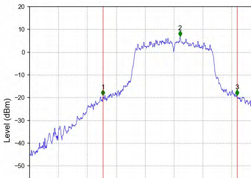
802.11a_MCH_5580MHz_Ant2_NTNV
