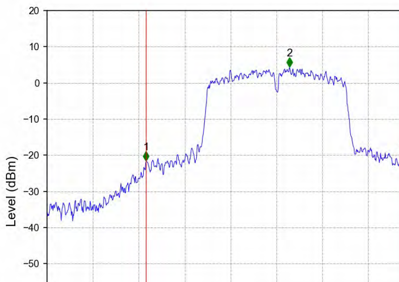
802.11n(HT40)_HCH_5230MHz_Ant2_NTNV
