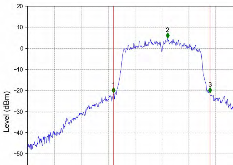
802.11n(HT20)_HCH_5700MHz_Ant2_NTNV
