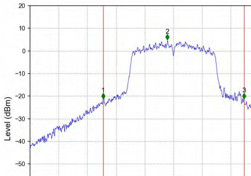
802.11n(HT20)_MCH_5300MHz_Ant2_NTNV
