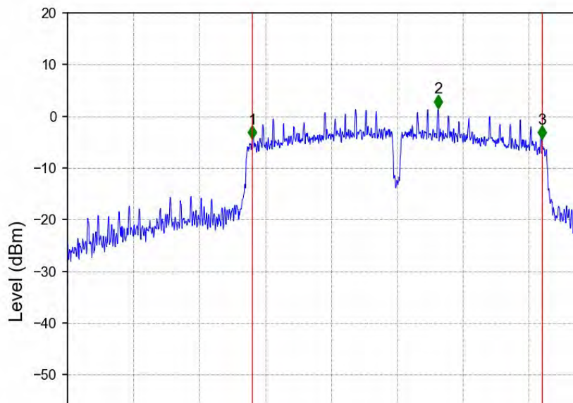
802.11n(HT40)_LCH_5755MHz_Ant2_NTNV
