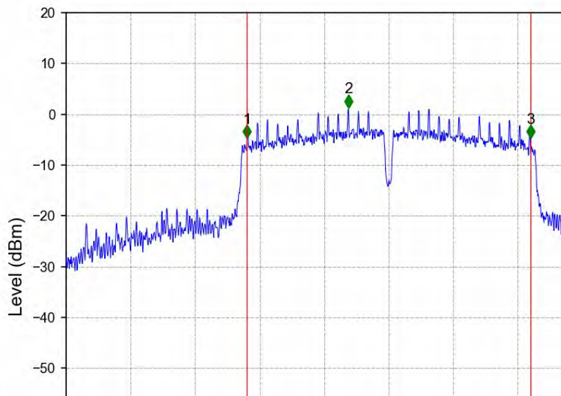
802.11n(HT40)_HCH_5795MHz_Ant2_NTNV
