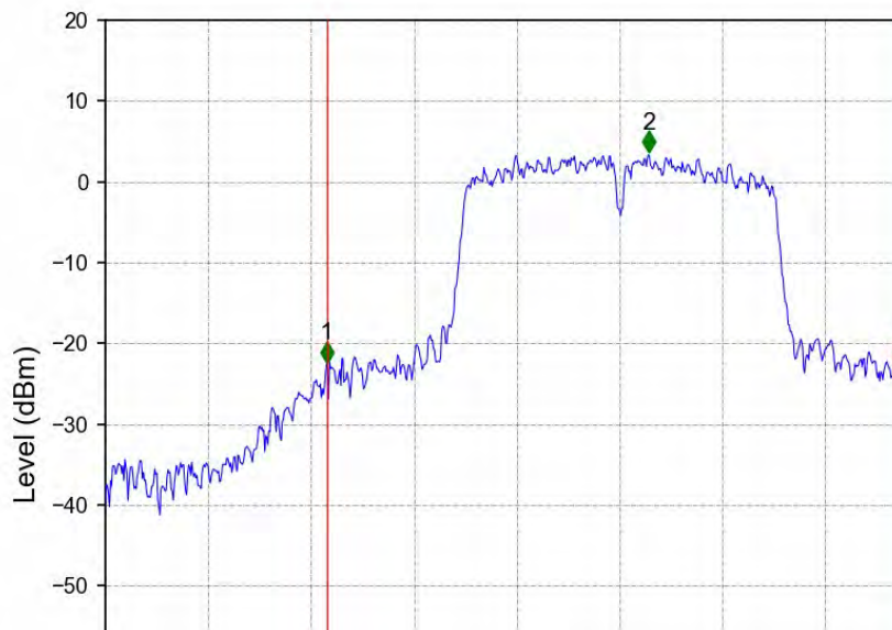
802.11n(HT40)_LCH_5190MHz_Ant2_NTNV
