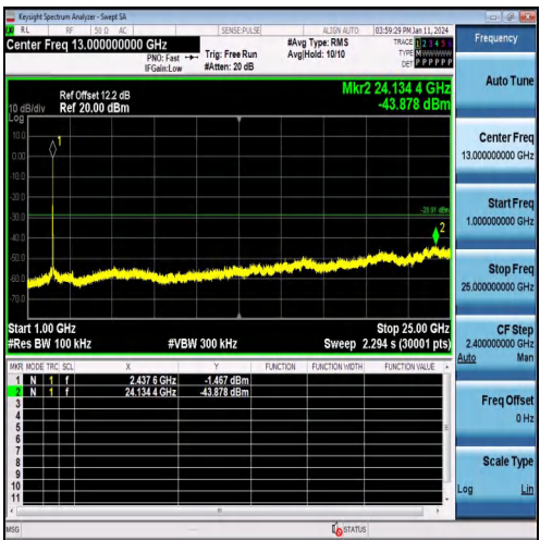
1GHz -25GHz
