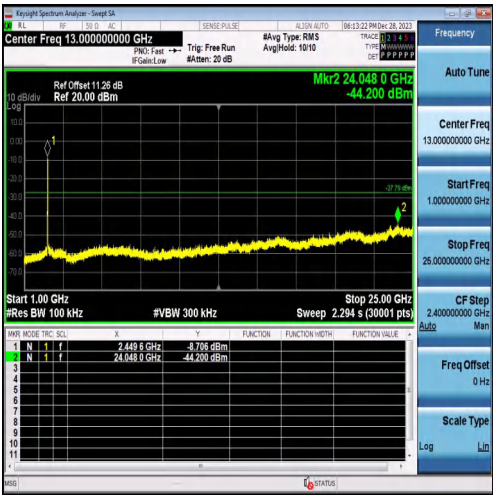
1GHz-25GHz
