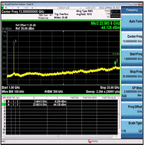
1GHz-25GHz
