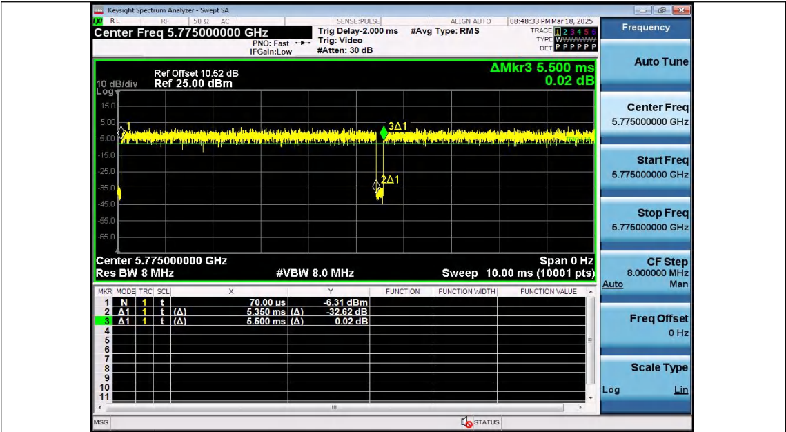
NTNV-11AC80SISO-Ant2-5775
