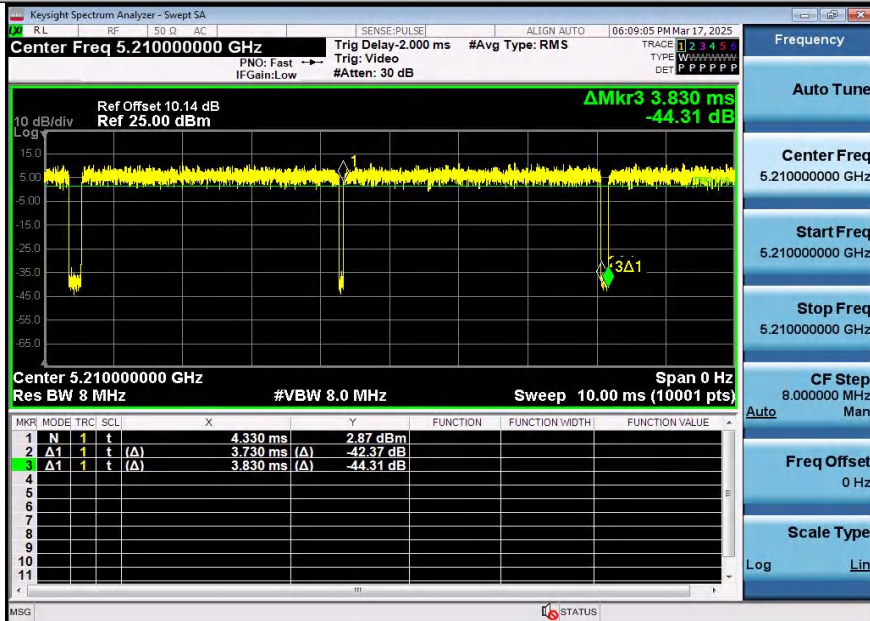
NTNV-11AX80SISO-Ant1-5210
