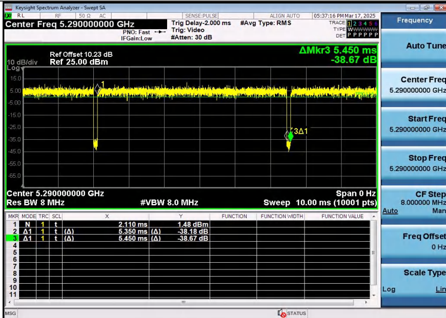
NTNV-11AC80SISO-Ant1-5290
