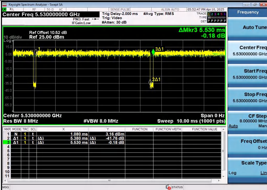
NTNV-11AX80SISO-Ant1-5530
