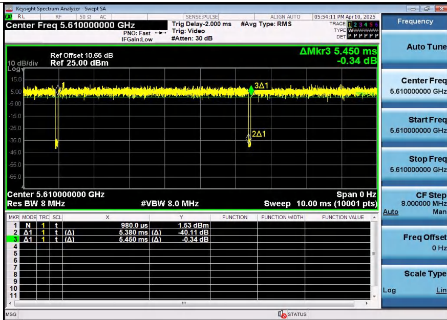
NTNV-11AX80SISO-Ant1-5610
