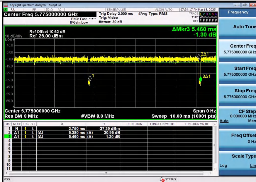
NTNV-11AX80SISO-Ant1-5775
