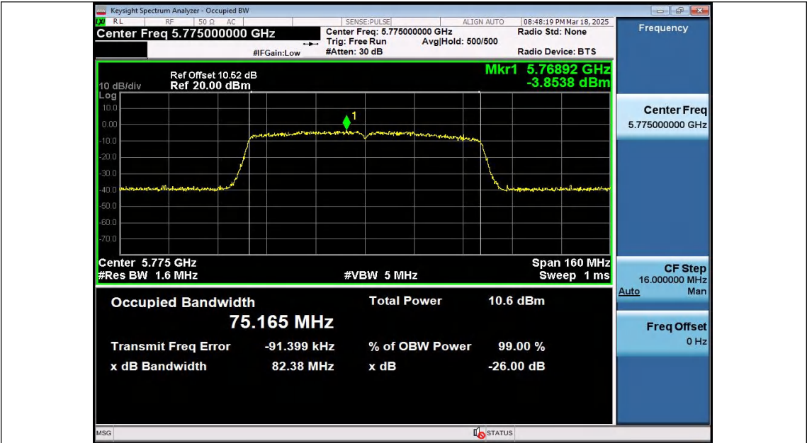
11AC80SISO-Ant2-5775
