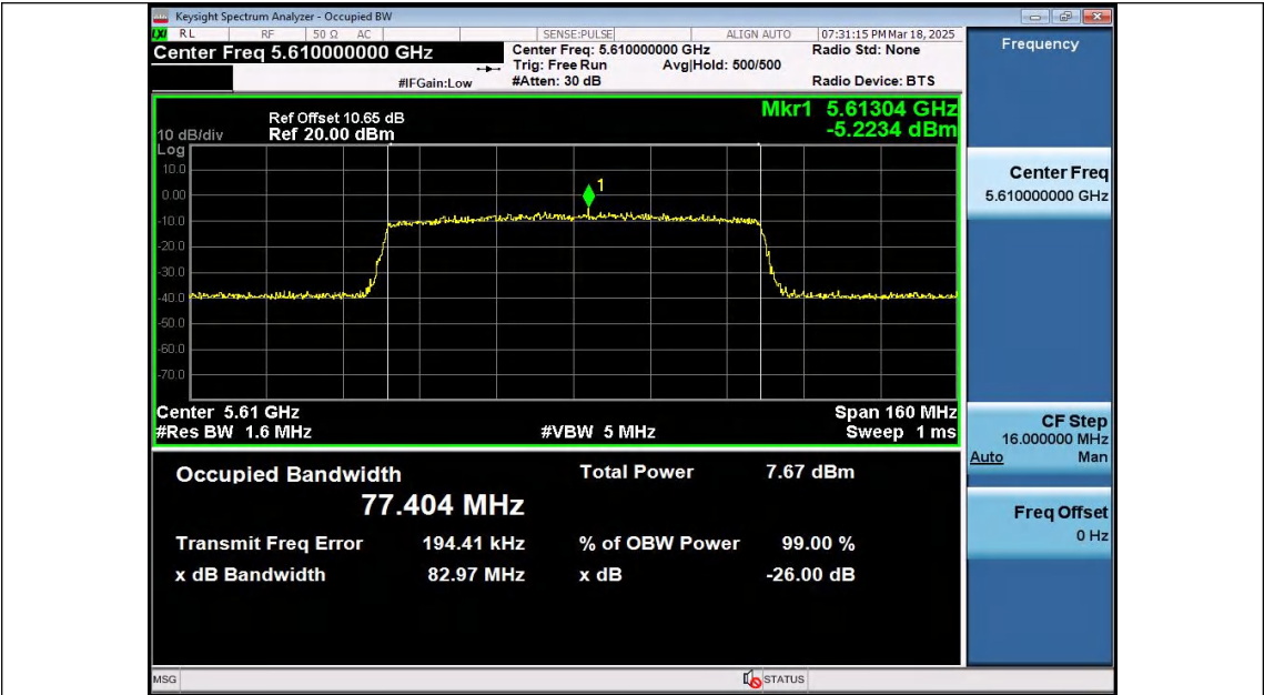
11AX80SISO-Ant1-5610
