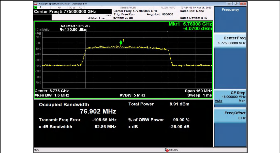
11AX80SISO-Ant1-5775
