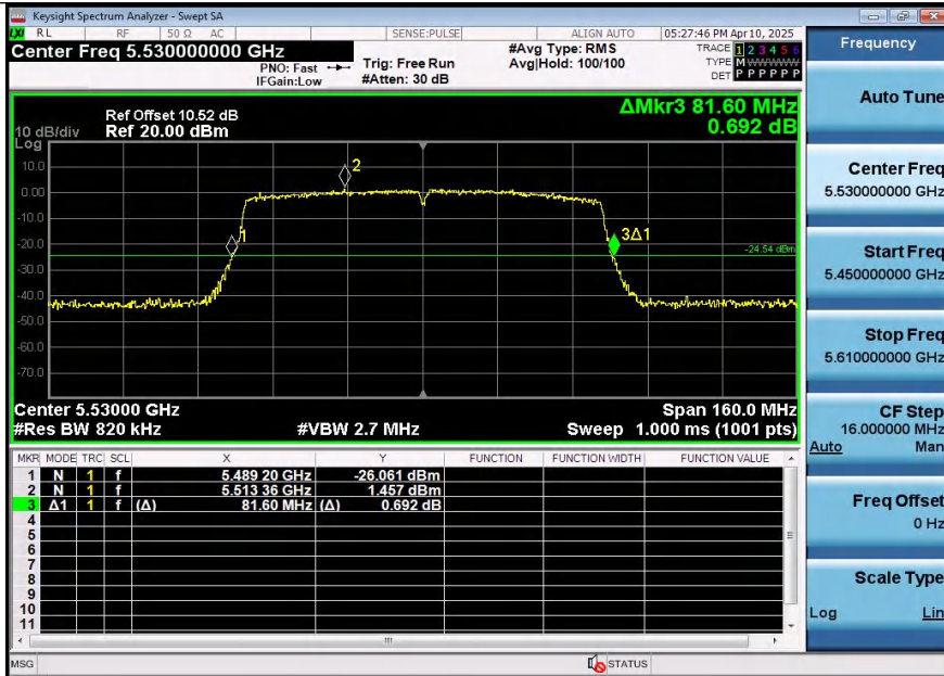
11AC80SISO-Ant1-5530
