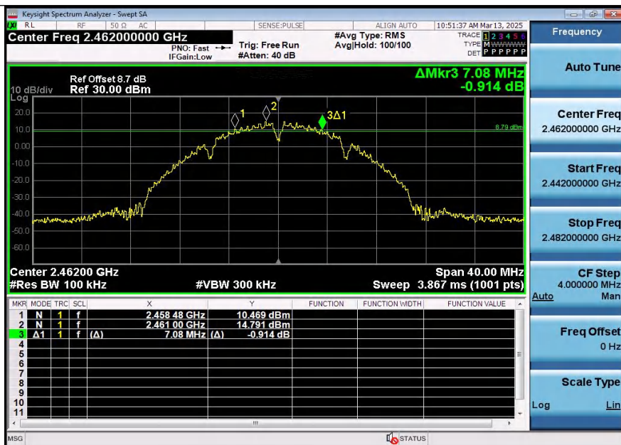
11B-Ant2-2462-PASS
