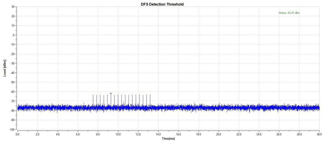
11N40-5510-Type3-PASS
