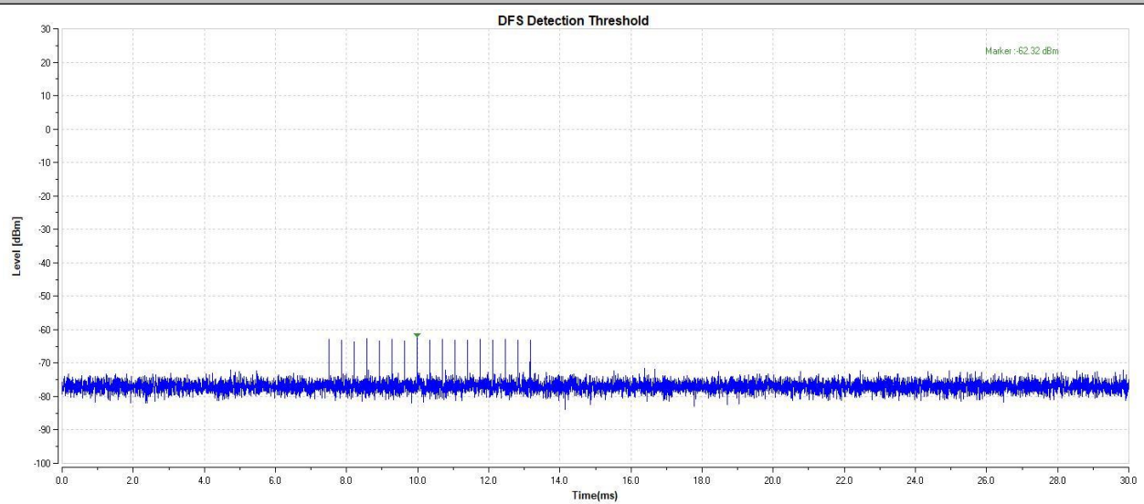
11N40-5270-Type3-PASS
