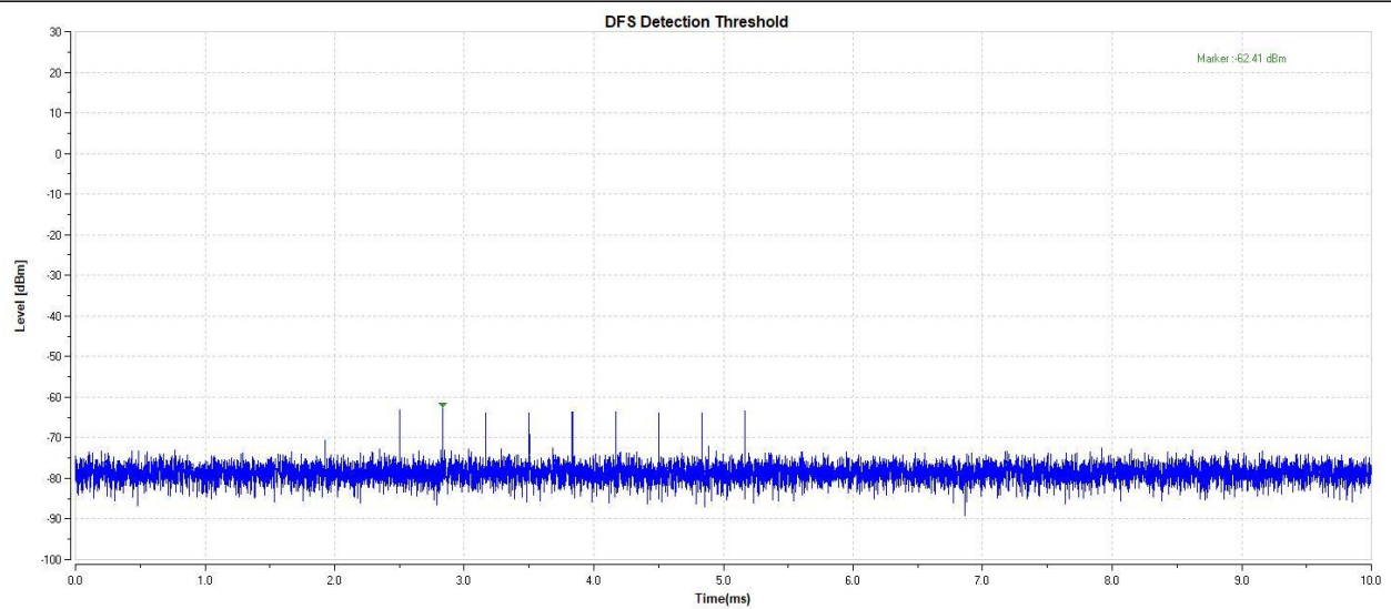
11N40-5270-Type6-PASS
