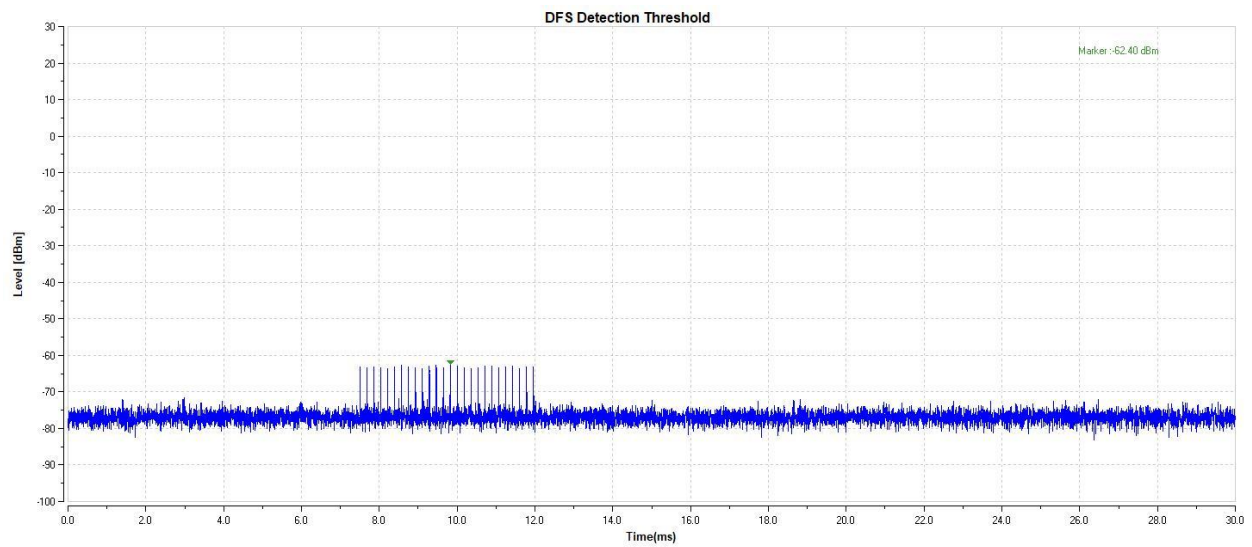
11N40-5270-Type2-PASS
