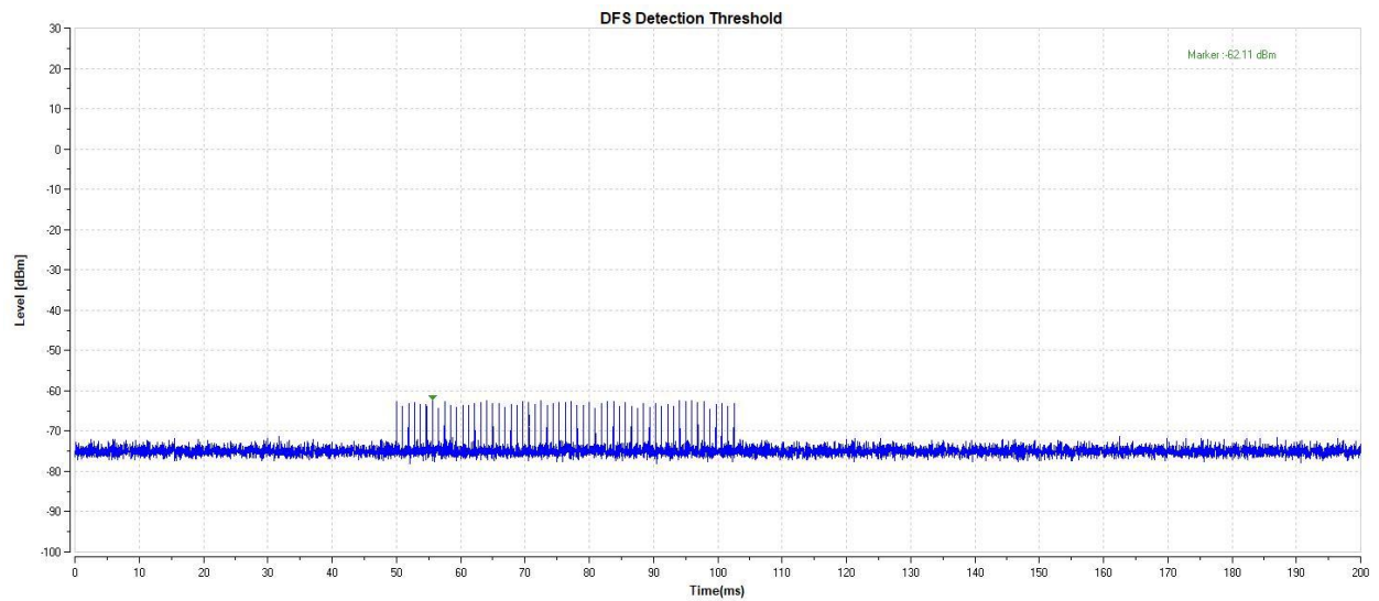
11N40-5270-Type1-PASS
