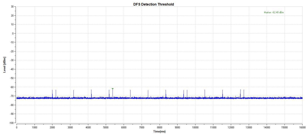
11N40-5270-Type5-PASS
