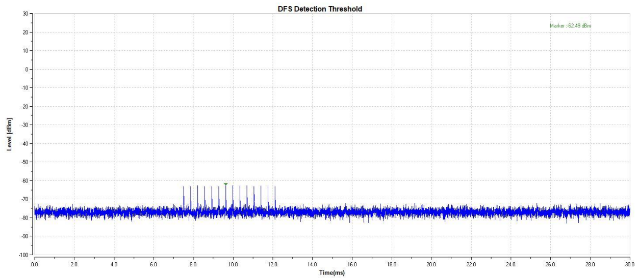
11N40-5510-Type4-PASS
