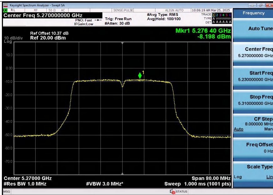
11N40SISO-Ant2-5270-PASS
