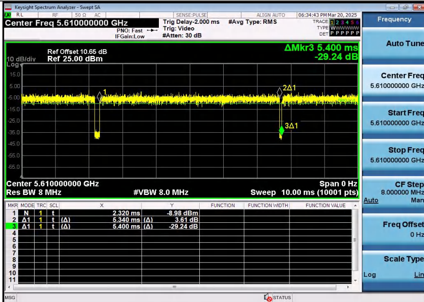
NTNV-11AC80SISO-Ant2-5610
