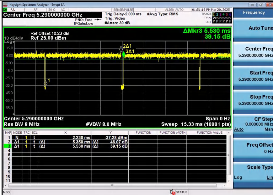
NTNV-11AC80SISO-Ant2-5290
