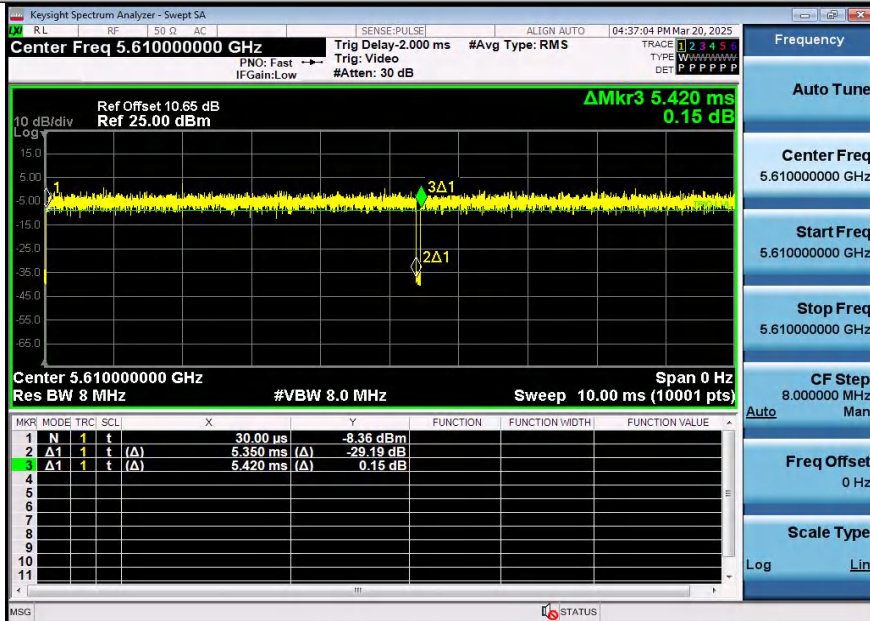
NTNV-11AC80SISO-Ant1-5610
