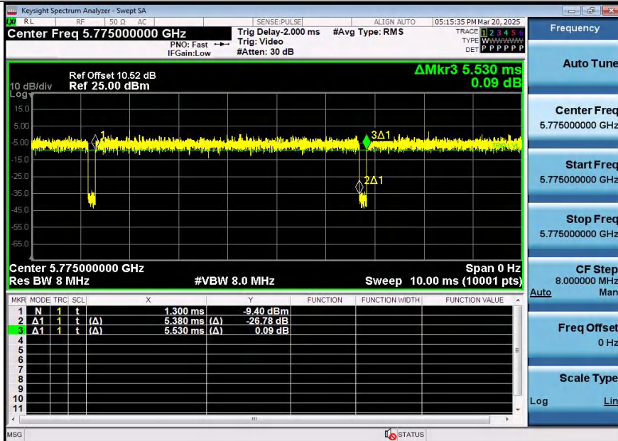
NTNV-11AX80SISO-Ant1-5775
