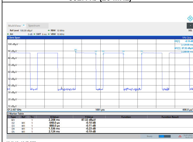
802.11b (20 MHz)
