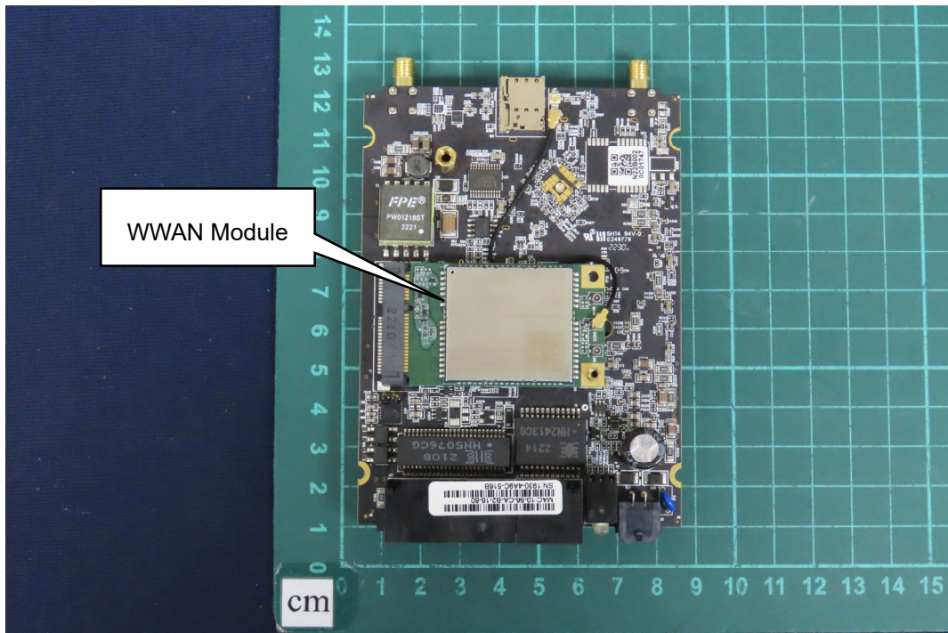
(4) EUT Photo
