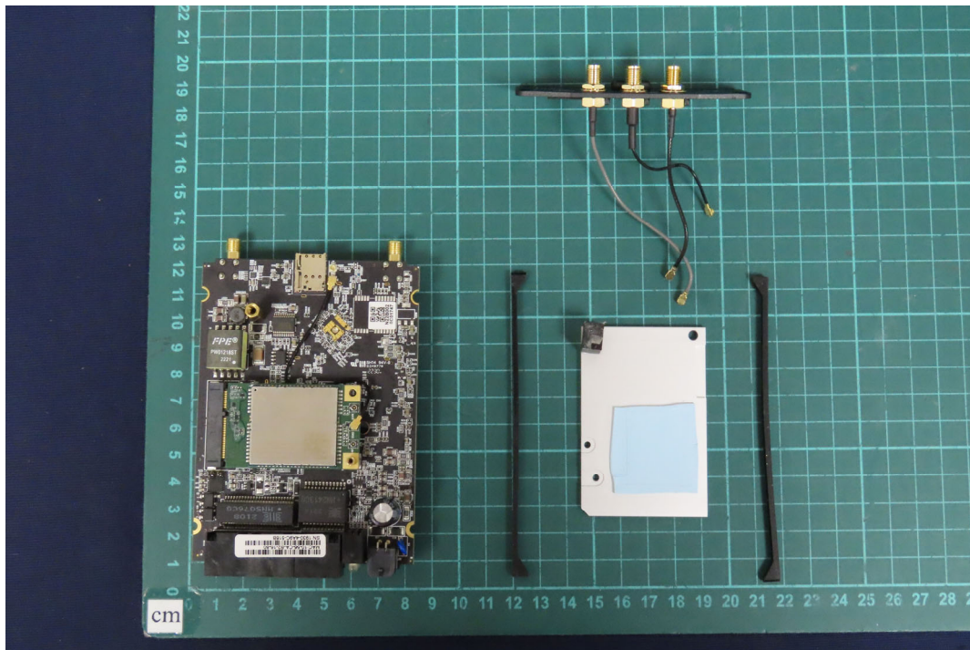
(3) EUT Photo
