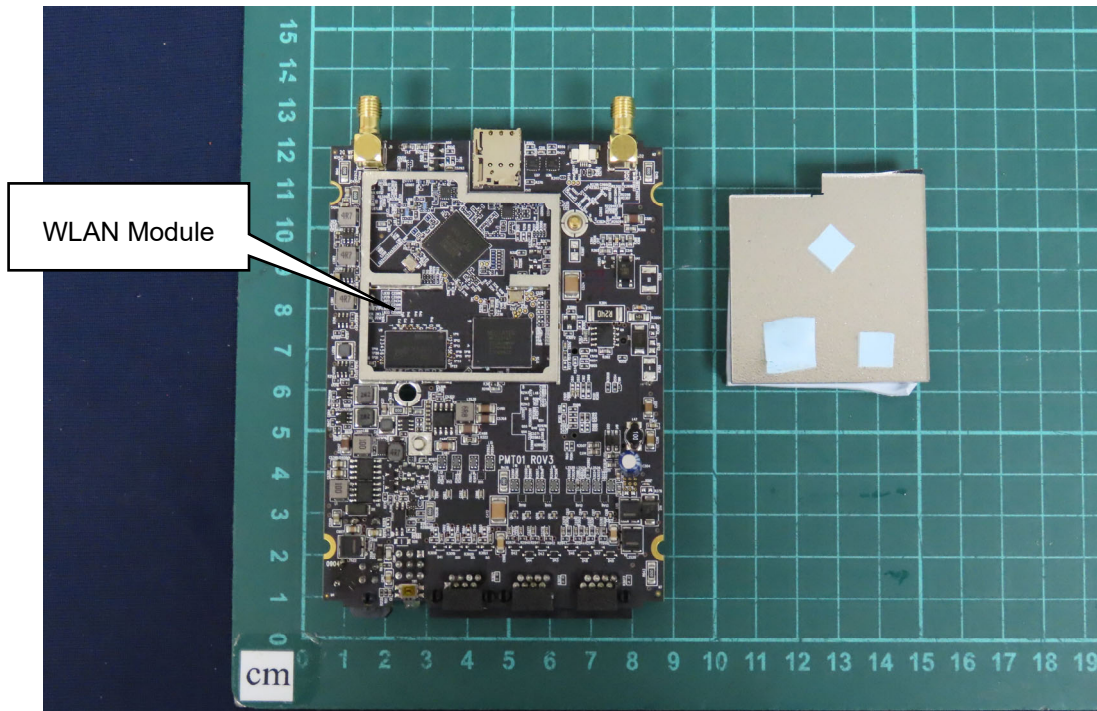
(10) EUT Photo
