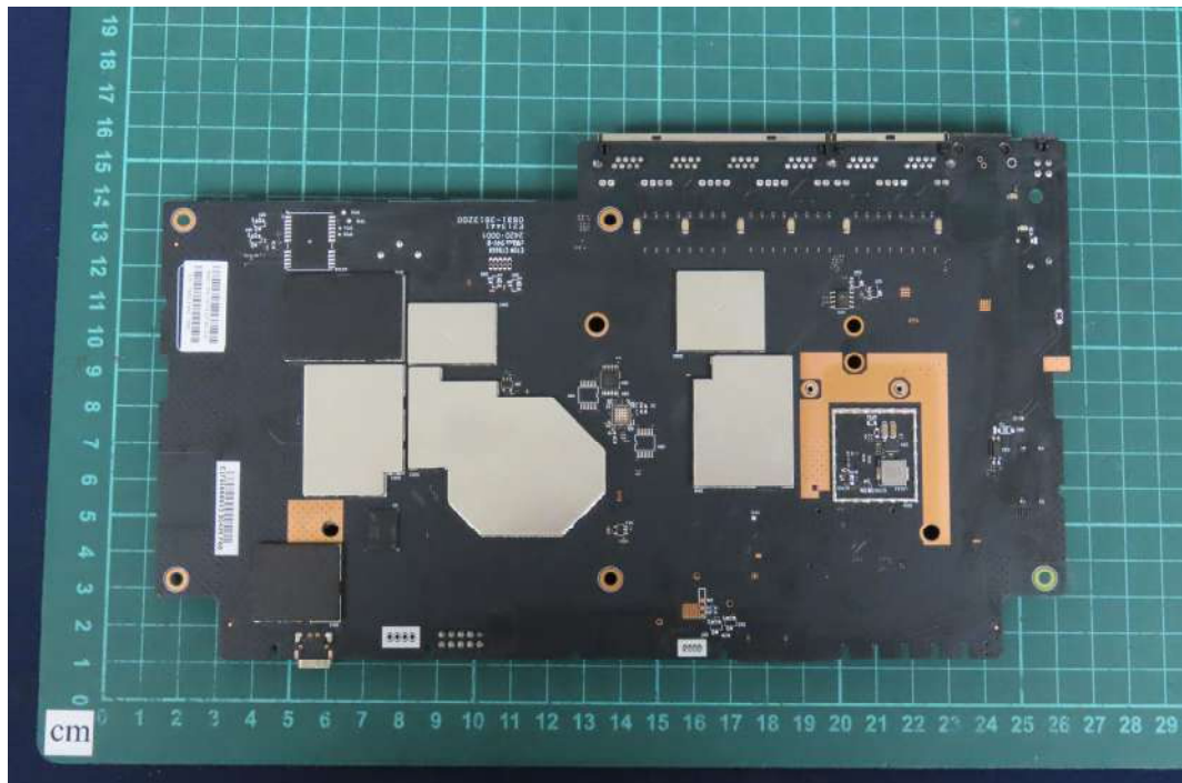
(46) EUT Photo
