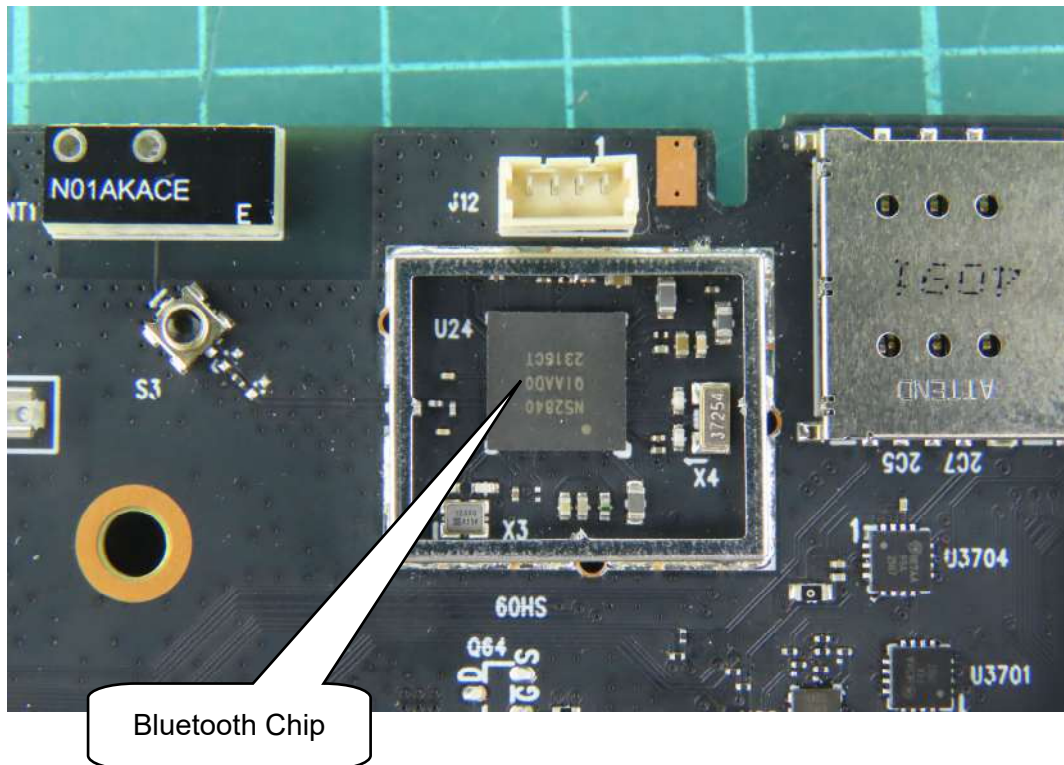
(40) EUT Photo
