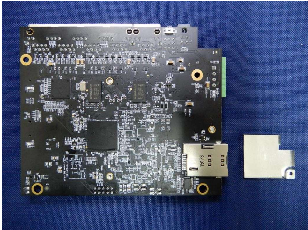
(13) EUT Photo
