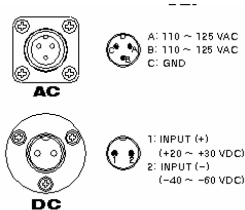
<Pic.4> AC & DC ports
