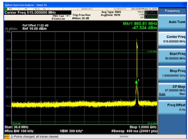
800 MHz band (30 MHz – 1 GHz) CDMA+LTE 5MHz
