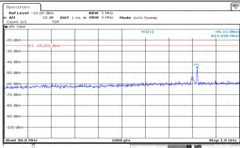
Band7-10MHz-QPSK-20800-50RB#0-Range1:30~1000MHz
