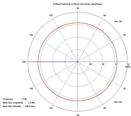
Azimuth (H-plane)
