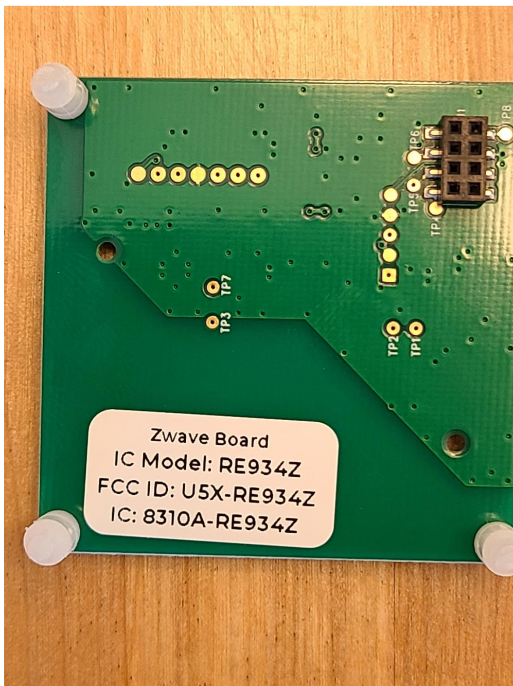
Zwave Module (rear side)
