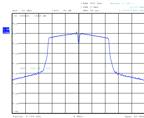
11N40SISO-Ant1-5755-PASS
