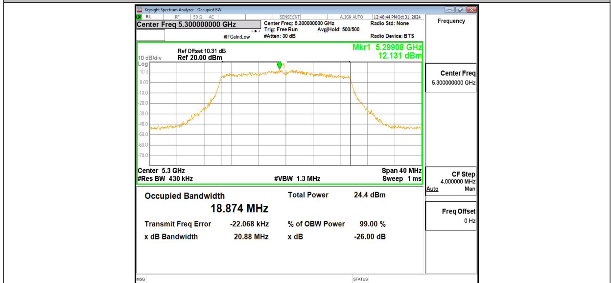
11AX20MIMO_Ant8_5300
