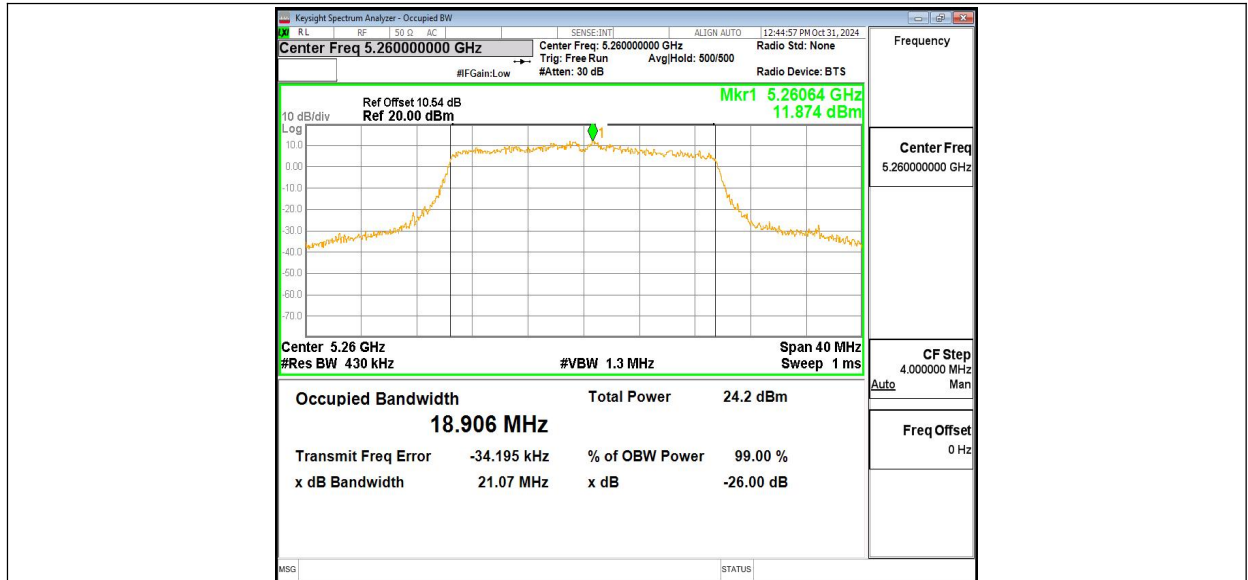
11AX20MIMO_Ant9_5260
