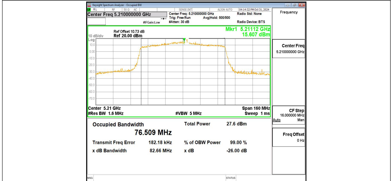
11AX80MIMO_Ant9_5210
