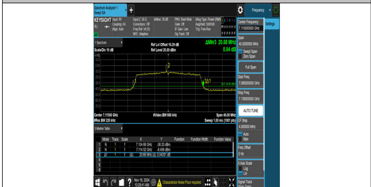
11AX20MIMO-Ant9-7115
