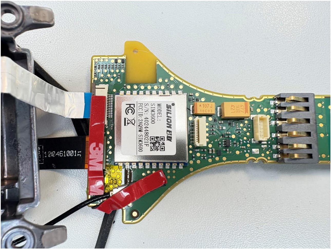
RFID Module
