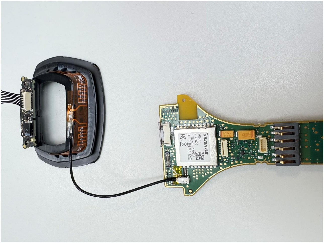
RFID module + antenna
