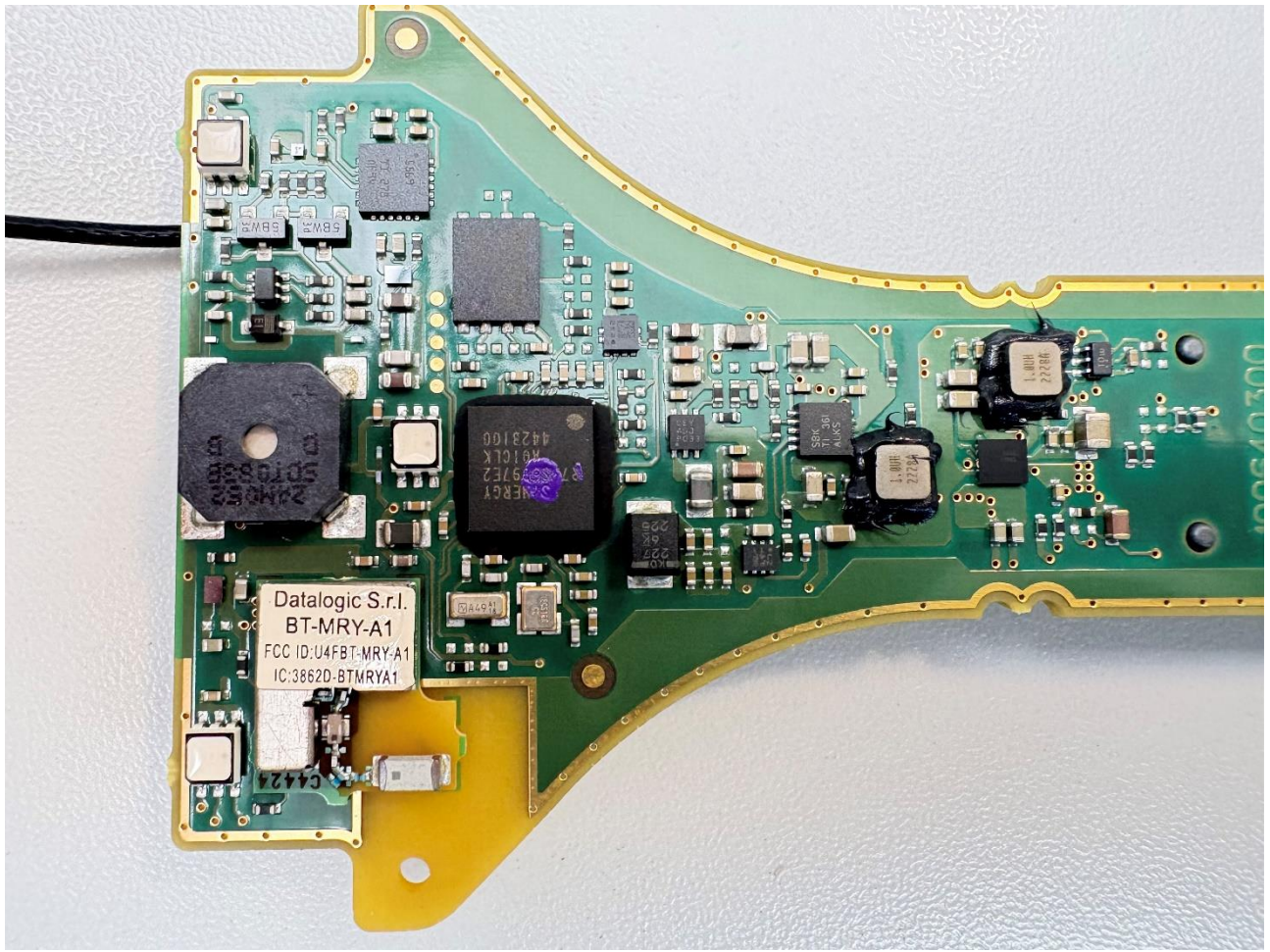
BT module
