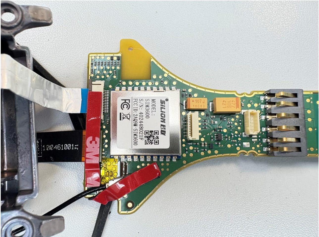
Antenna
