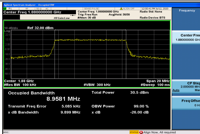
Band2-10MHz-16QAM-18900-50RB#0-8.9581
