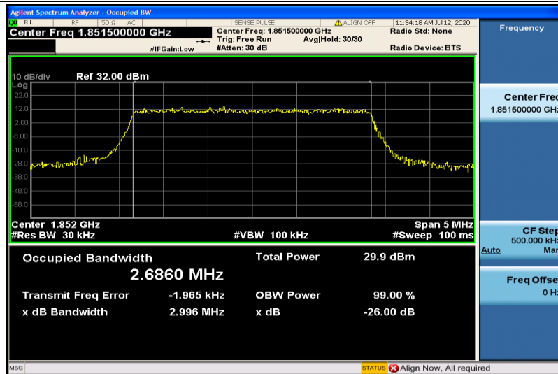
Band2-3MHz-16QAM-18615-15RB#0-2.6860
