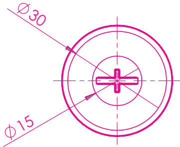
LABEL DIMENSIONS
