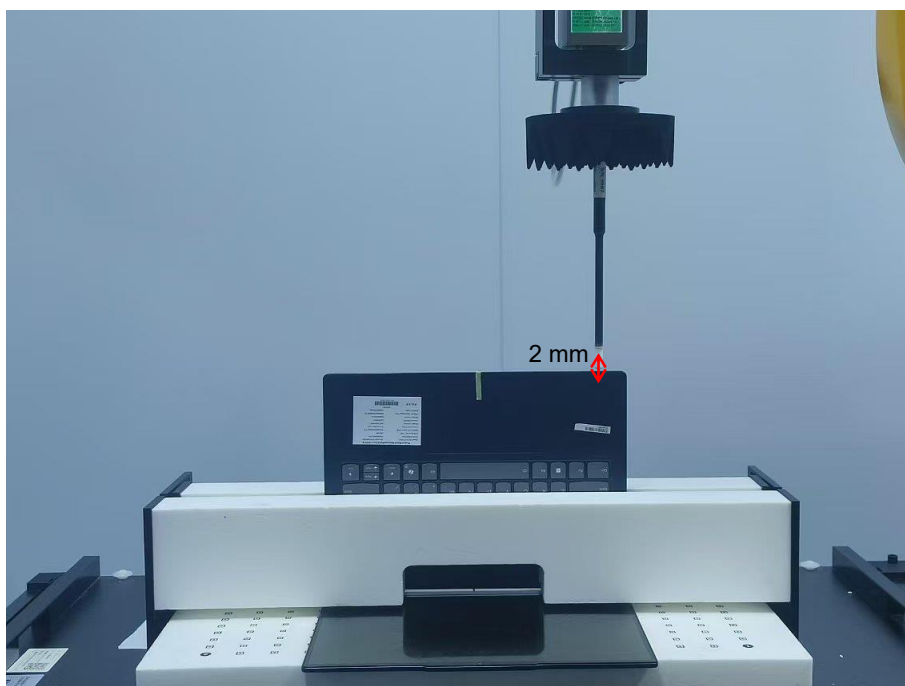
Front Edge (Laptop) (2mm)
