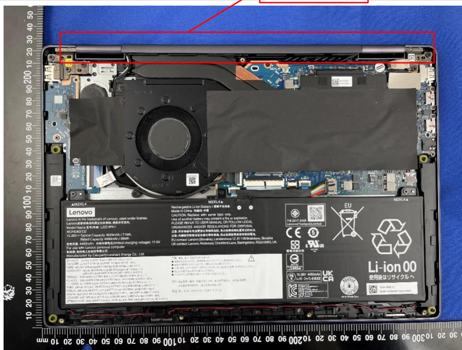
PIFA Antenna
